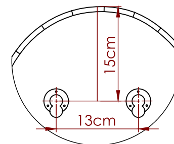
DETALHE A ESCALA 1 : 5
